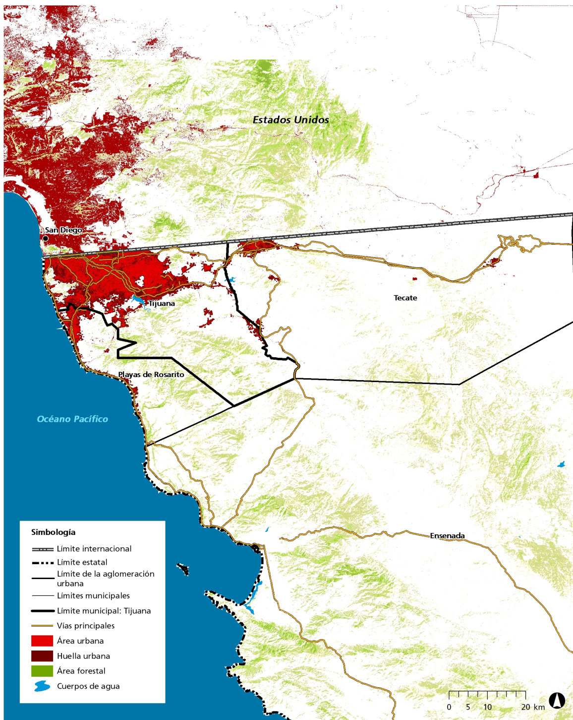
MAPA 2 • Delimitación de la aglomeración urbana de Tijuana
